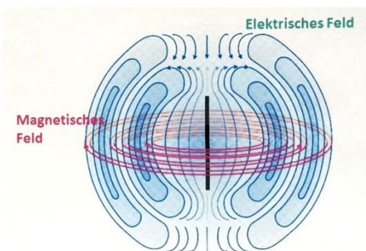
Folie 9 zur Abstrahlung der Sendeantenne
