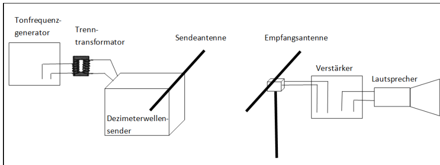
Abb. 1: Schematischer Aufbau des Demonstrationsversuchs zur Informationsübertragung
